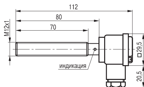
Габаритный чертеж
