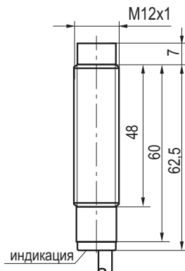
Габаритный чертеж
