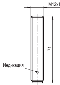
Габаритный чертеж
