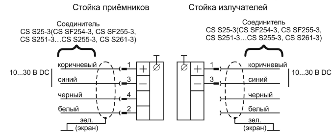
Цоколёвка разъемов Вид на розетку соединителя со стороны подключения
