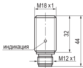
Габаритный чертеж
