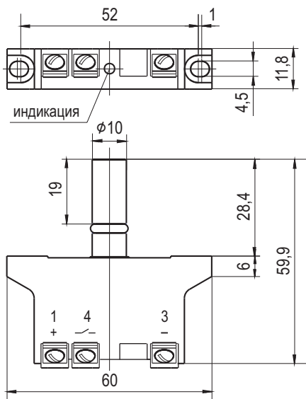
Габаритный чертеж
