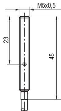
Габаритный чертеж
