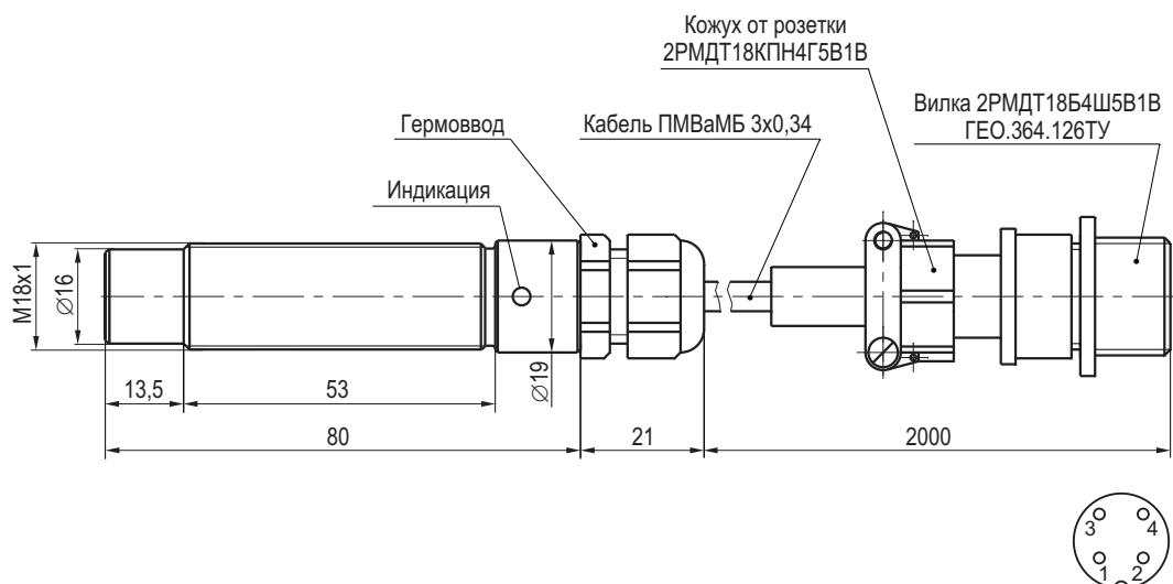
Габаритный чертеж
