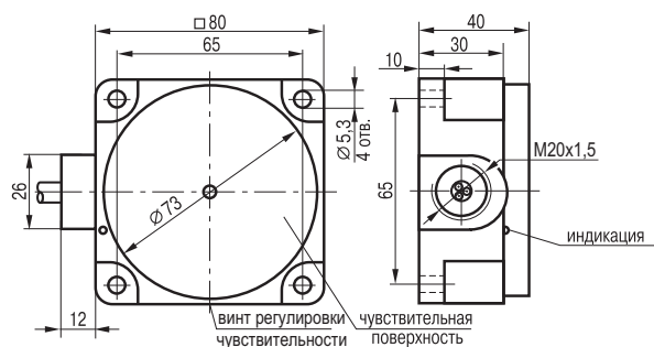
Габаритный чертеж
