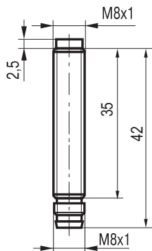
Габаритный чертеж
