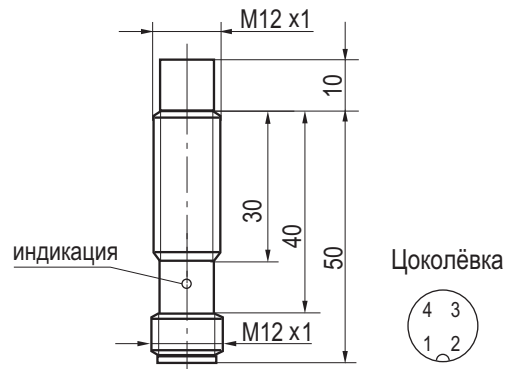
Габаритный чертеж
