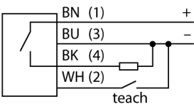
Схема подключения
