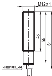
Габаритный чертеж
