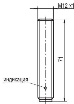
Габаритный чертеж
