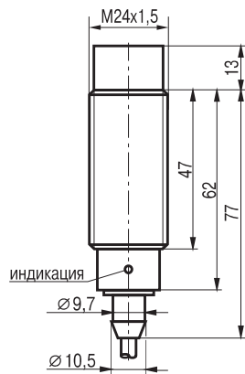
Габаритный чертеж
