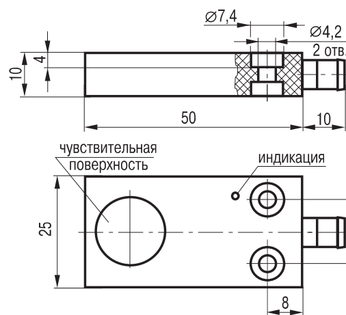
Габаритный чертеж
