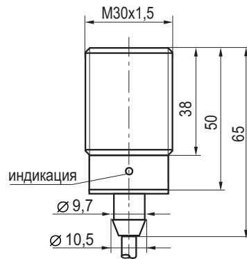
Габаритный чертеж
