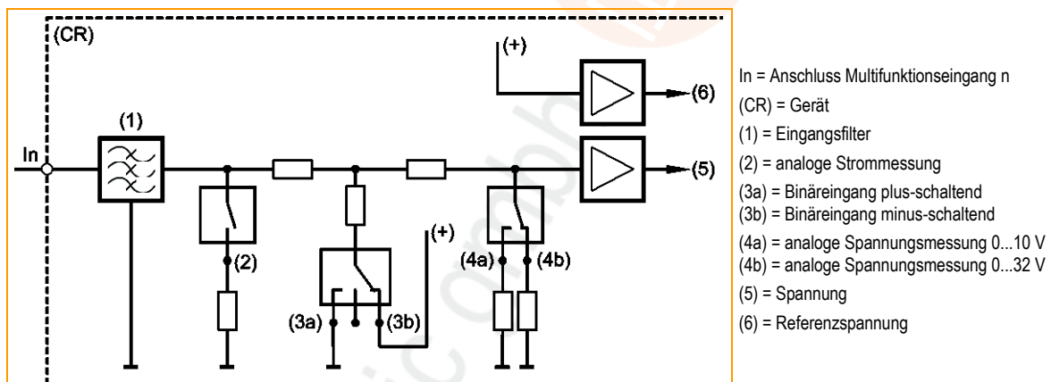
Grafik: Prinzipischiung Multifunktionseingang
