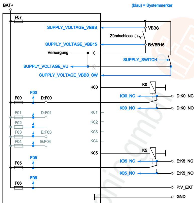
Grafik: Prinzipaufbau der Versorgung und der Relais
