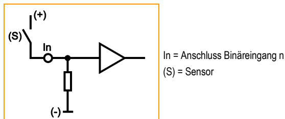
Prinzipischiung Binäreingang plus-schaltend (BL) für positives Sensorsignal: Eingang = offen \Rightarrow Signal = Low (GND)
