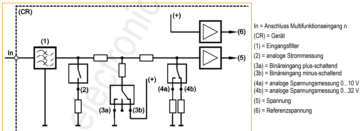
Grafik: Prinzipschaltung Multifunktionseingang
