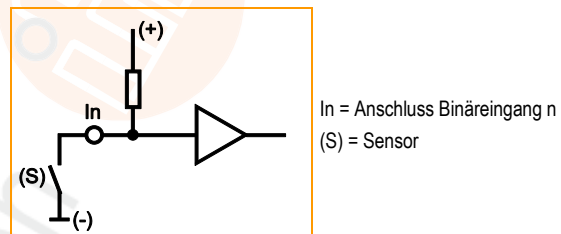
Prinzipischiung Binäreingang minus-schaltend (BH) für negatives Sensorsignal: Eingang = offen \Rightarrow Signal = High (Supply)
