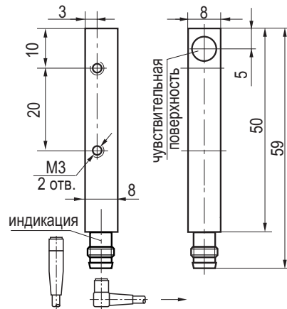
Габаритный чертеж
