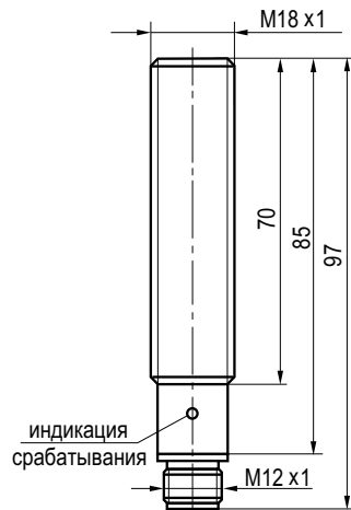
Габаритный чертеж.
