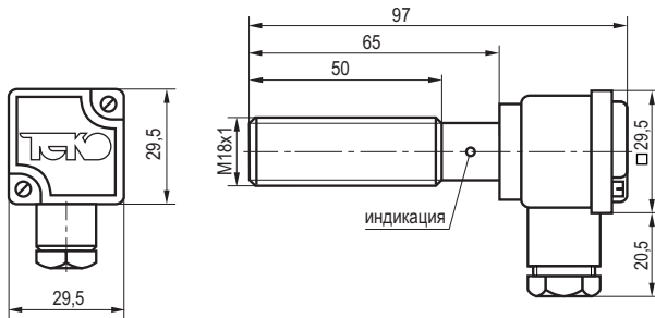
Габаритный чертеж
