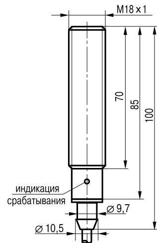
Габаритный чертеж.
