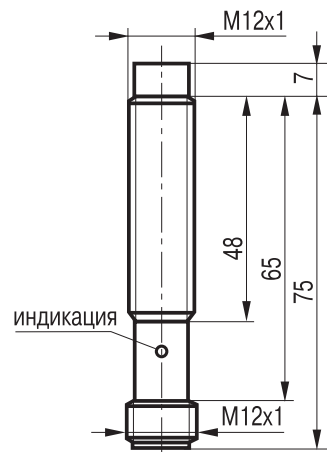
Габаритный чертеж
