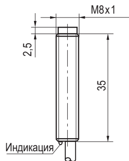
Габаритный чертеж
