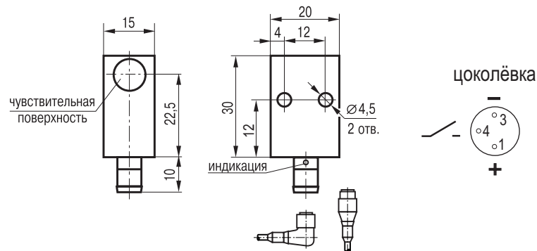
Габаритный чертеж
