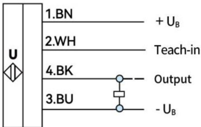
Аналоговый выход
