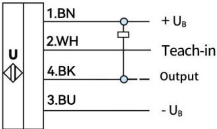
NPN
