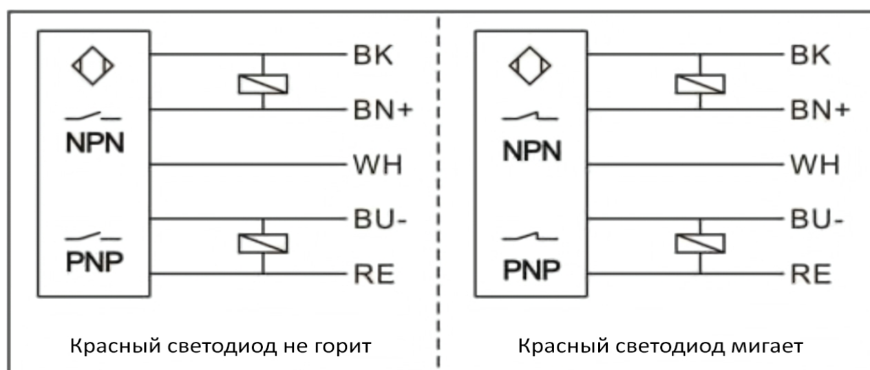
Схема подключения
