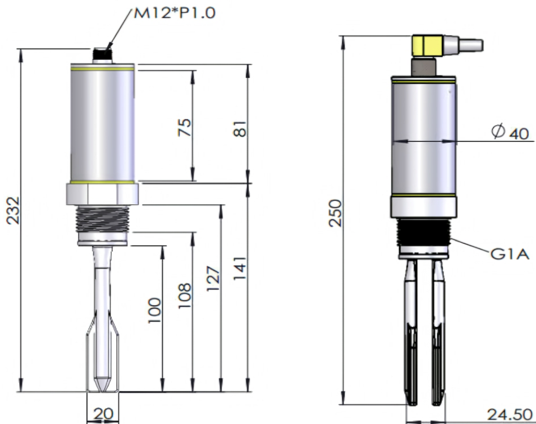
Размеры, мм
