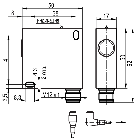
Габаритный чертеж
