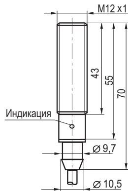
Габаритный чертеж
