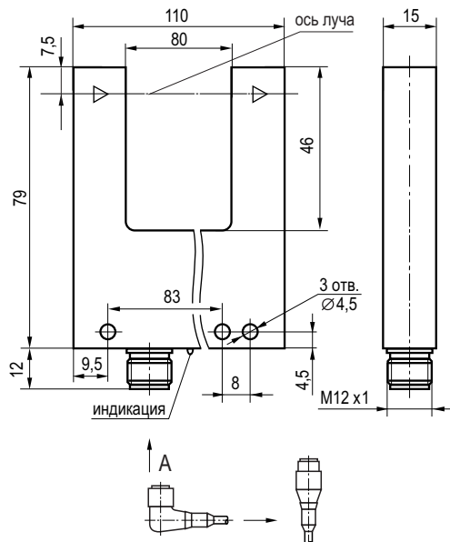
Габаритный чертеж
