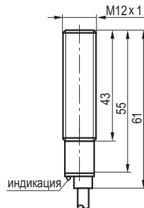
Габаритный чертеж
