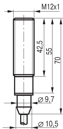
Габаритный чертеж
