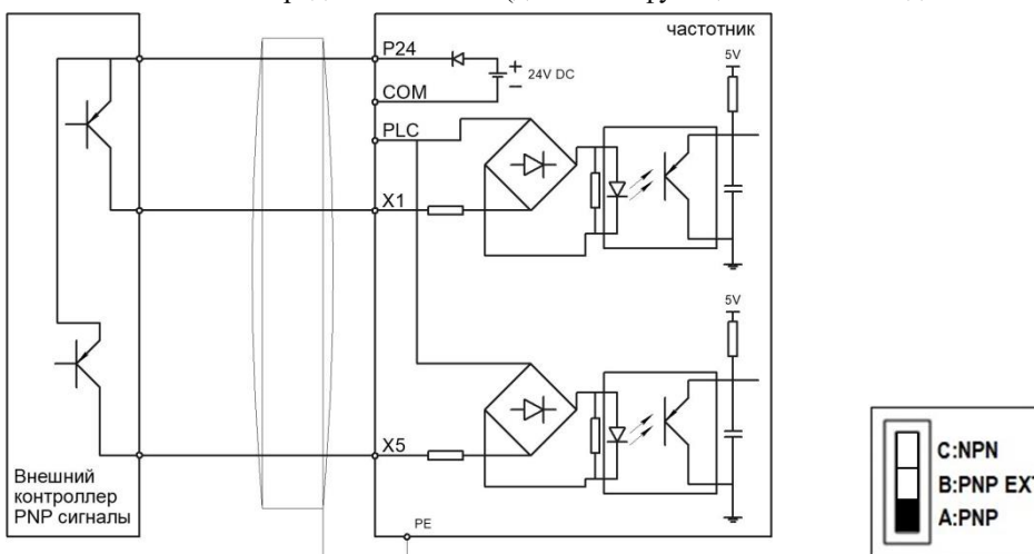
Рис. 3-15 Стандартный способ подключения PNP с внутренним источником питания 24VDC
