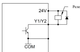
Рис. 3-16 Способ подключения внутреннего источника питания +24 В
