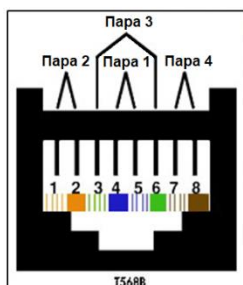
Рис. 3-19 Стандартный T568B
