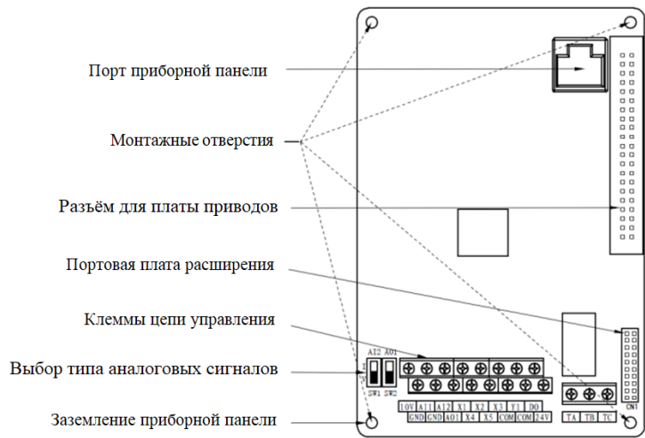
Рис. 3-20 Плата управления
