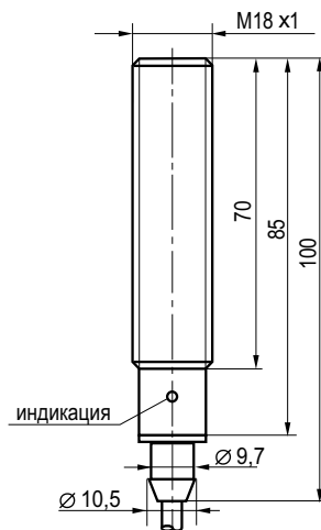
Габаритный чертеж
