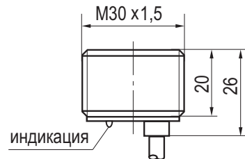
Габаритный чертеж
