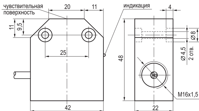
Габаритный чертеж
