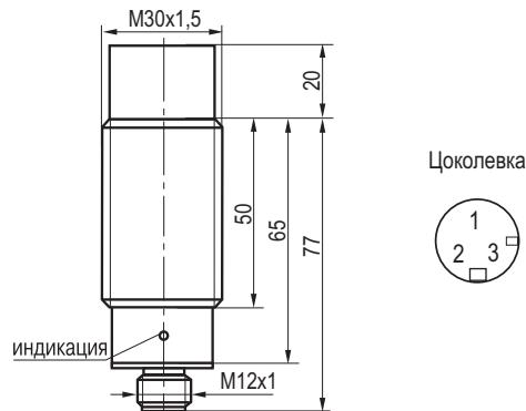
Габаритный чертеж
