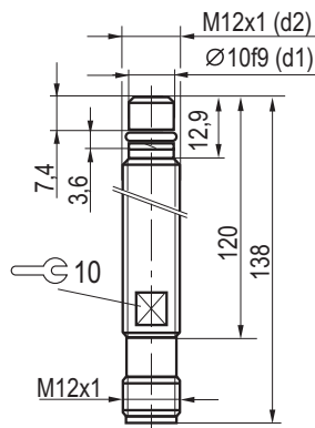
Схема монтажа
