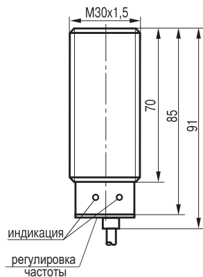
Габаритный чертеж
