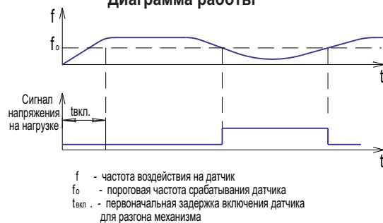
Диаграмма работы
