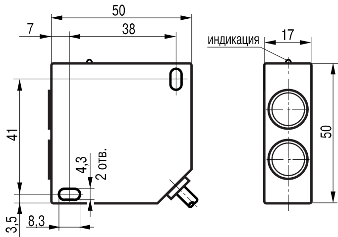
Габаритный чертеж.
