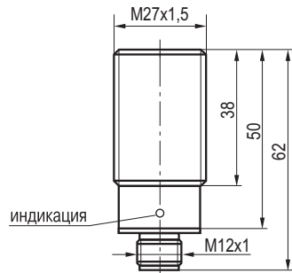
Габаритный чертеж
