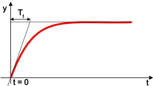
图：PT1 的时间特性
