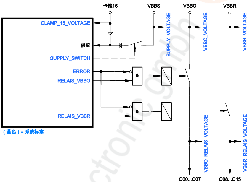
图：电源和继电器原理方块图
