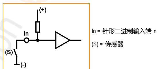
二进制输入端负极开关 (BH) 基本电路
