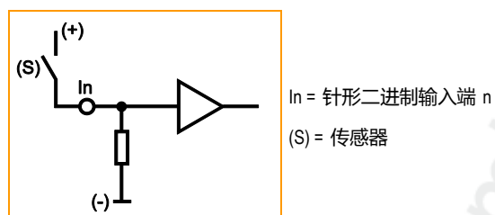
二进制输入端正极开关 (BL) 基本电路
