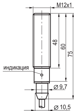
Габаритный чертеж
