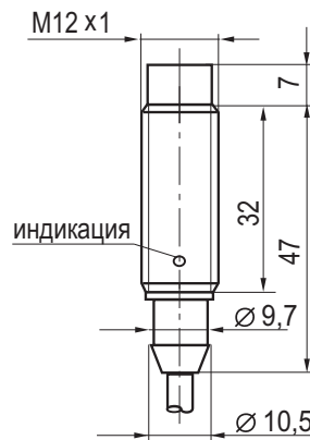
Габаритный чертеж
