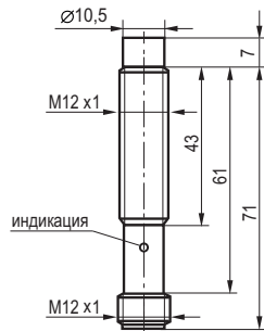
Габаритный чертеж
