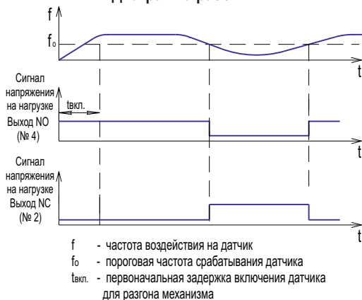
Диаграмма работы
