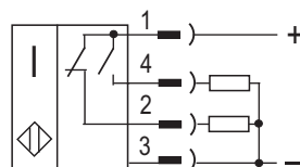
Схема подключения активной нагрузки
