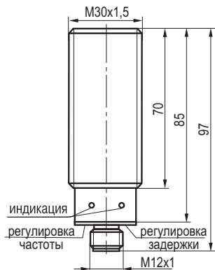
Габаритный чертеж
