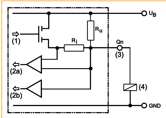
Grafik: Prinzipschaltung
