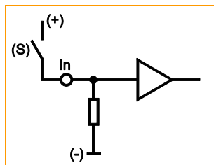
Prinzipischialtung Binäreingang plus-schaltend (BL) für positives Sensorsignal: Eingang = offen \Rightarrow Signal = Low (GND)
