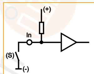
Prinzipischialtung Binäreingang minus-schaltend (BH) für negatives Sensorsignal: Eingang = offen \Rightarrow Signal = High (Supply)
