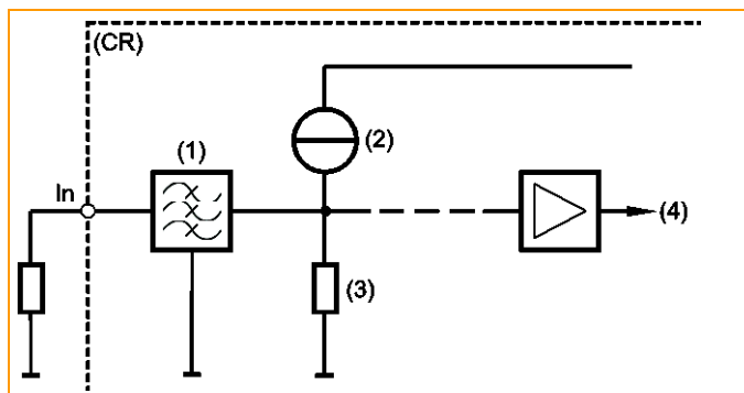
Grafik: Prinzipschaltung Widerstandsmess-Eingang
