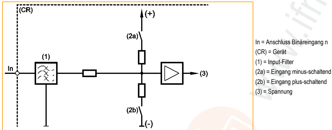
Grafik: Prinzipschialtung Binäreingang minus-schaltend / plus-schaltend für negative und positive Gebersignale
