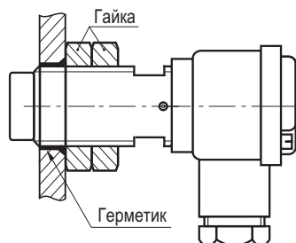
Схема монтажа
