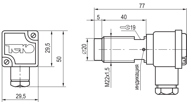
Схема монтажа
