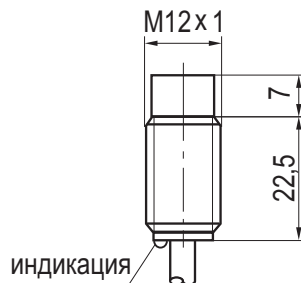
Габаритный чертеж
