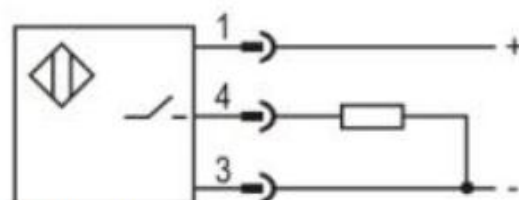
PNP NO
